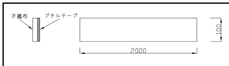
製品図
