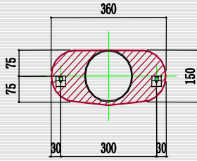
【外観図】
