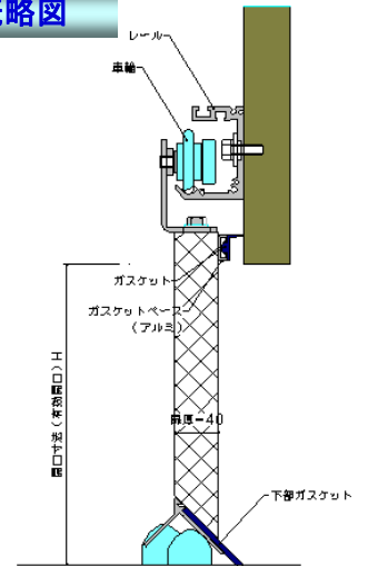
断面図
